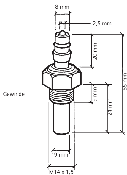
Spezial-Steckanschluss
